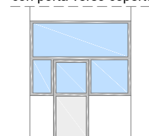
Particolare vetrata C-C' con porta verso copertura
