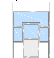
Particolare vetrata A-A' con porta verso balcone
